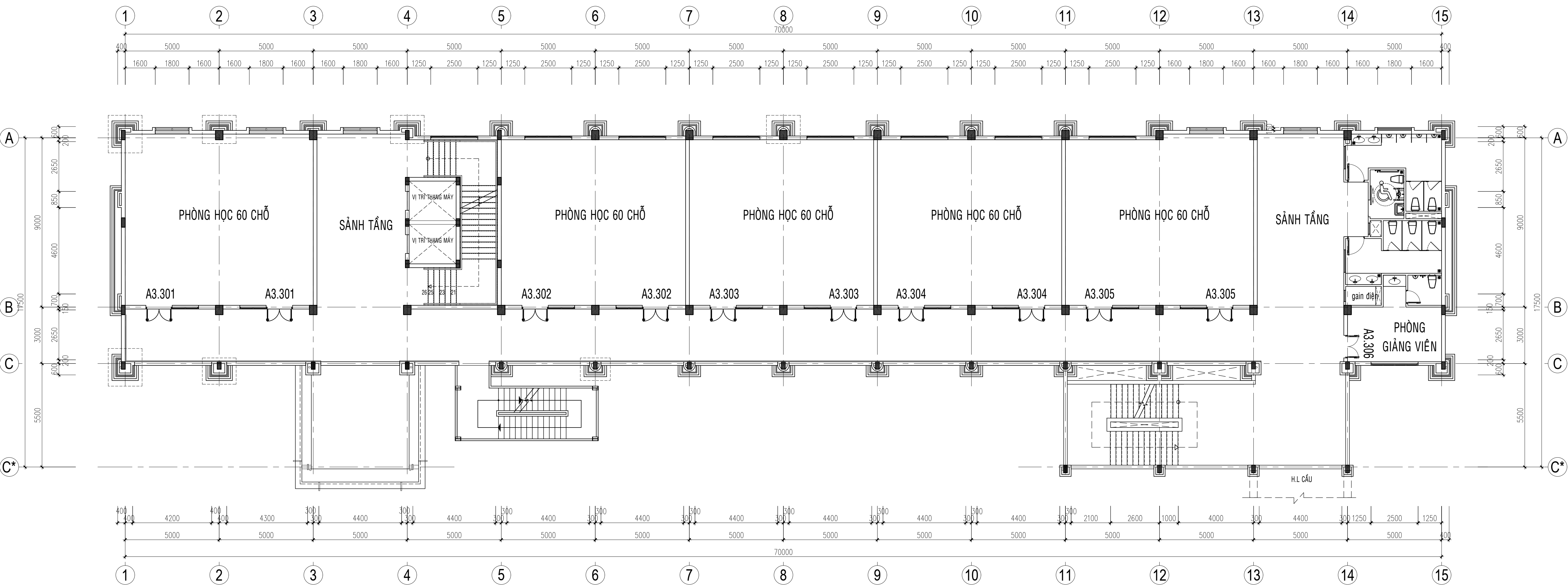
MẶT BẰNG BỐ TRÍ PHÒNG TẦNG 3
