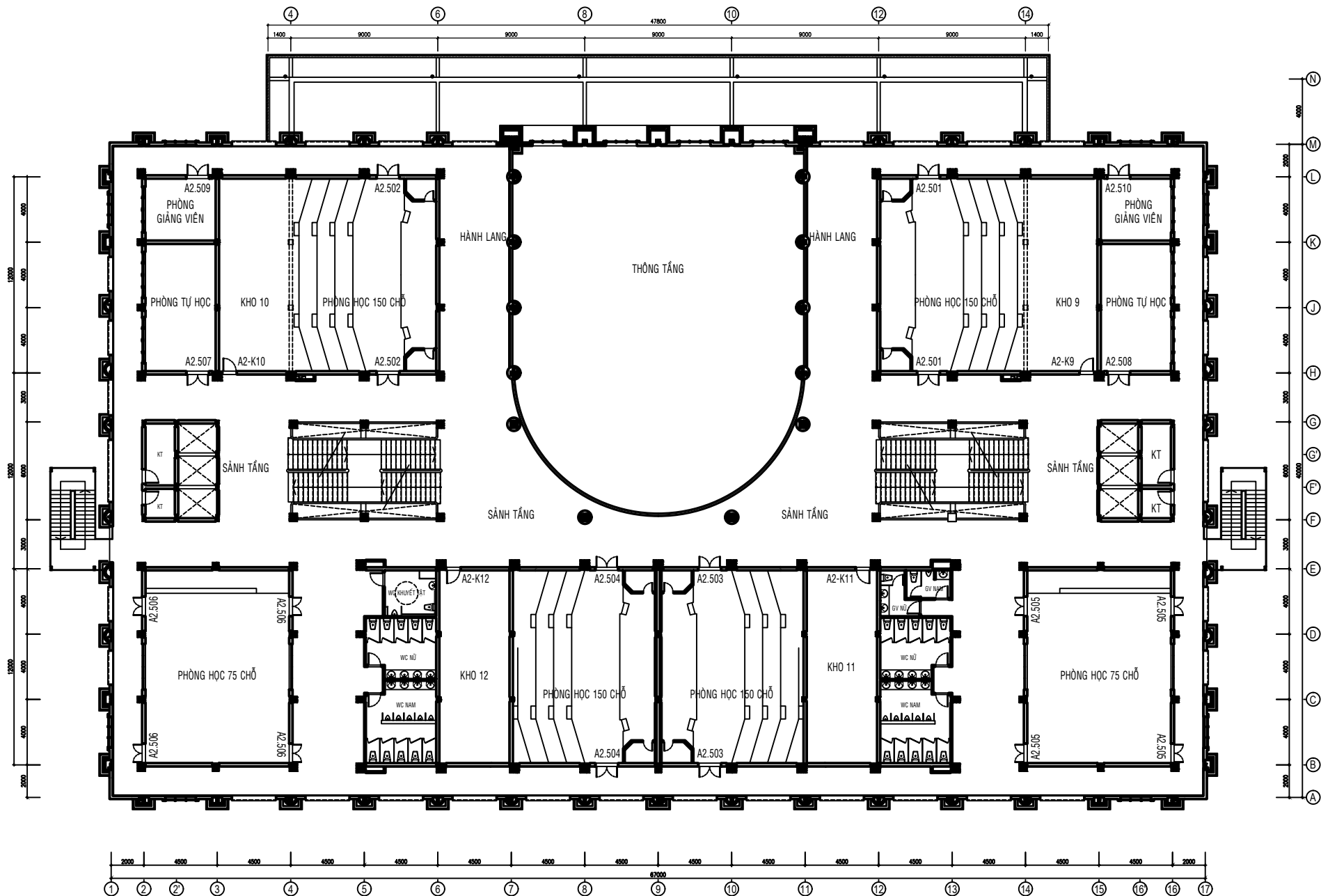
MẶT BẰNG BỐ TRÍ PHÒNG TẦNG 5 (TỶ LỆ: 1/100)
