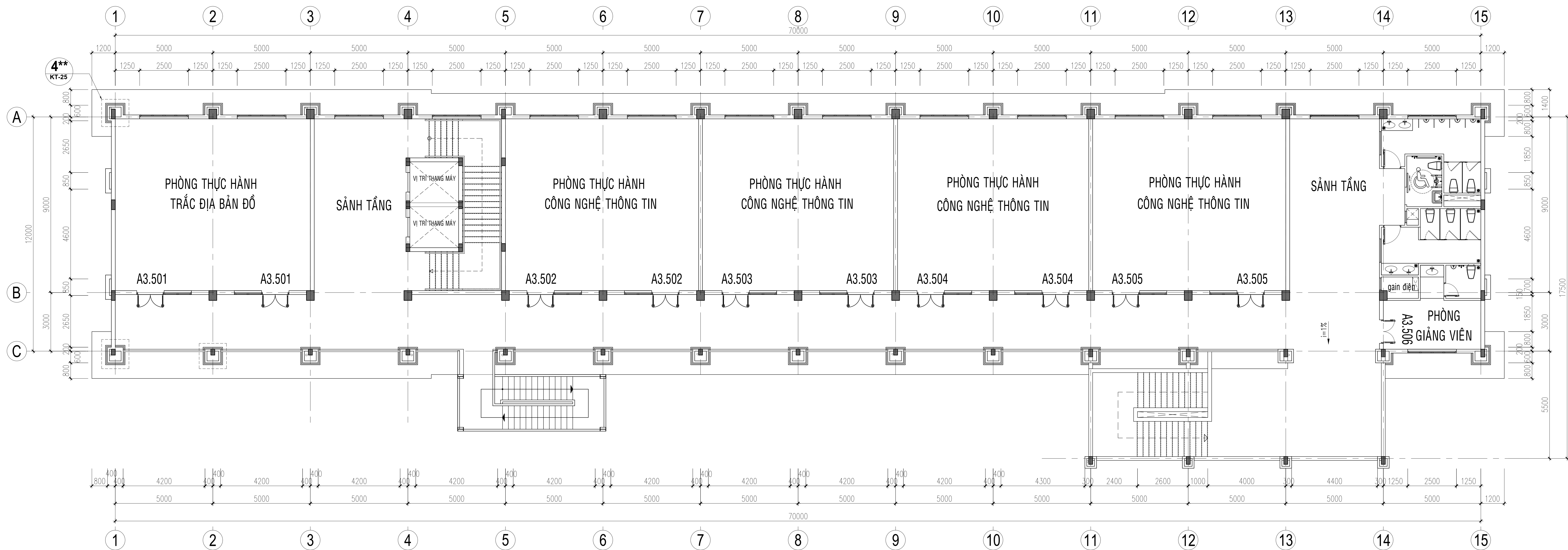
MẶT BẰNG BỐ TRÍ PHÒNG TẦNG 5
