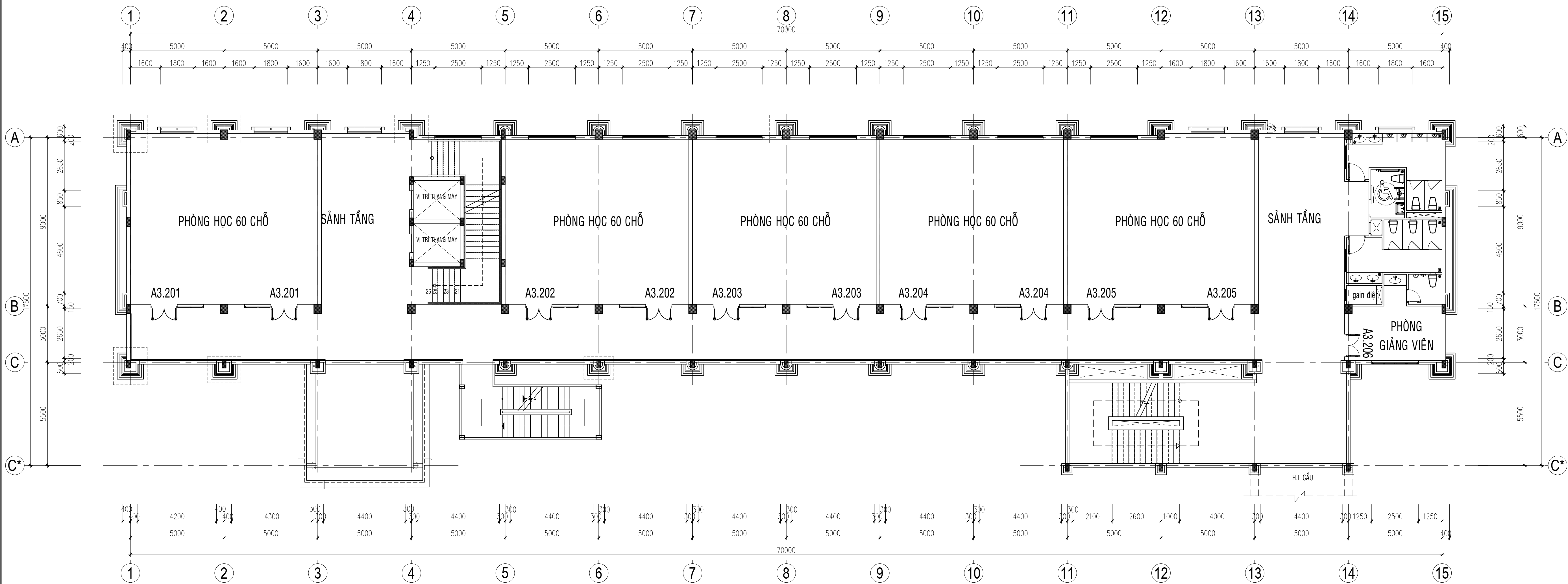
MẶT BẰNG BỐ TRÍ PHÒNG TẦNG 2
