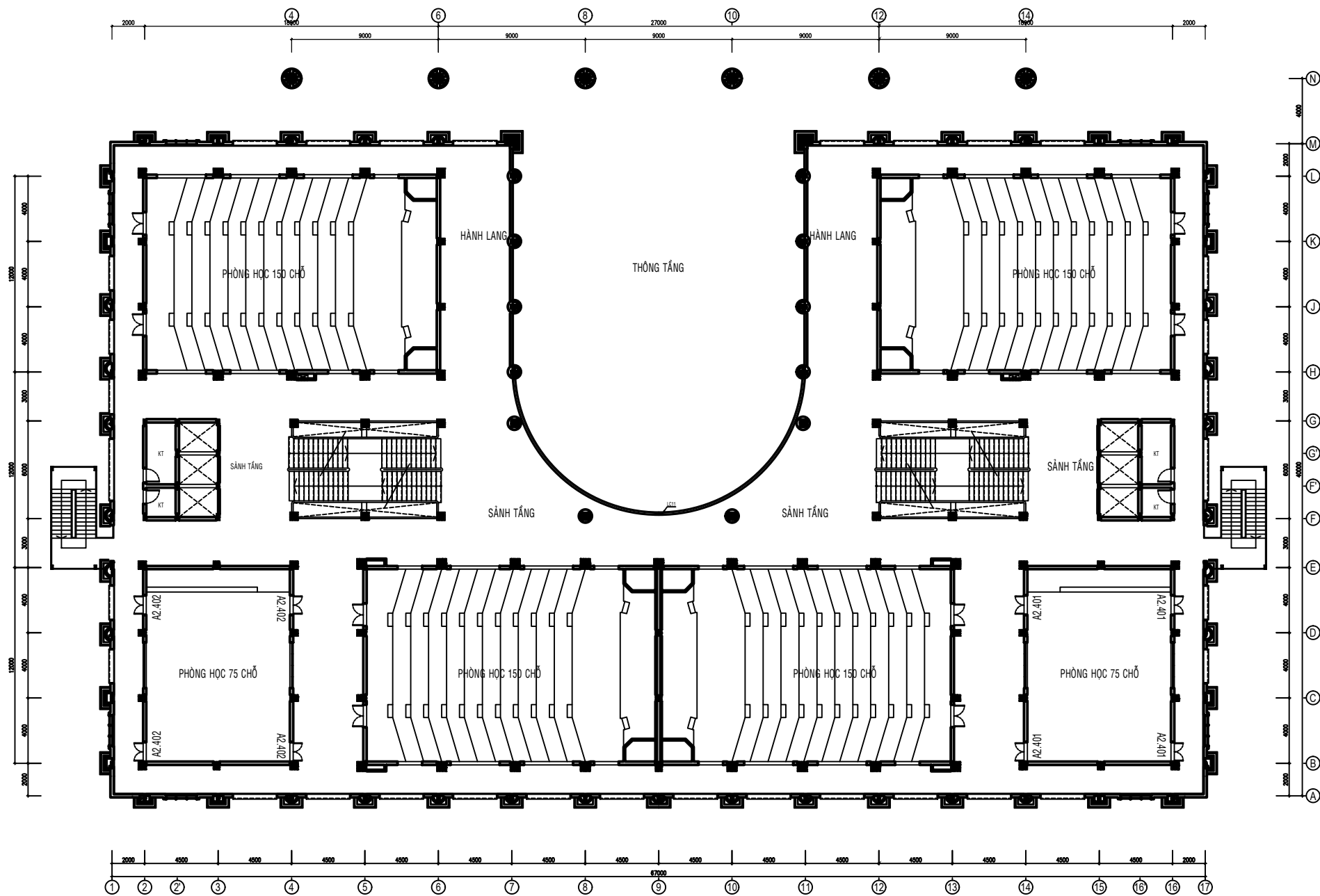
MẶT BẰNG BỐ TRÍ PHÒNG TẦNG 4 (TỶ LỆ: 1/100)
