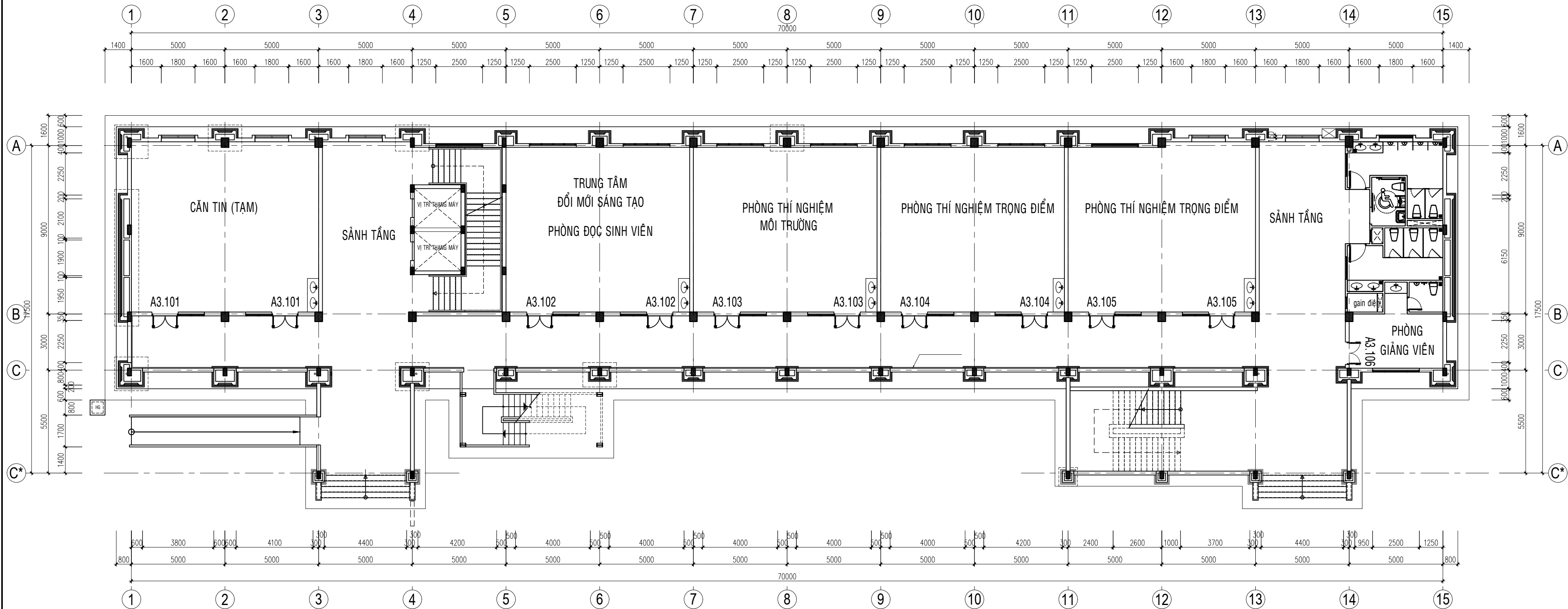
MẶT BẰNG BỐ TRÍ PHÒNG TẦNG 1
