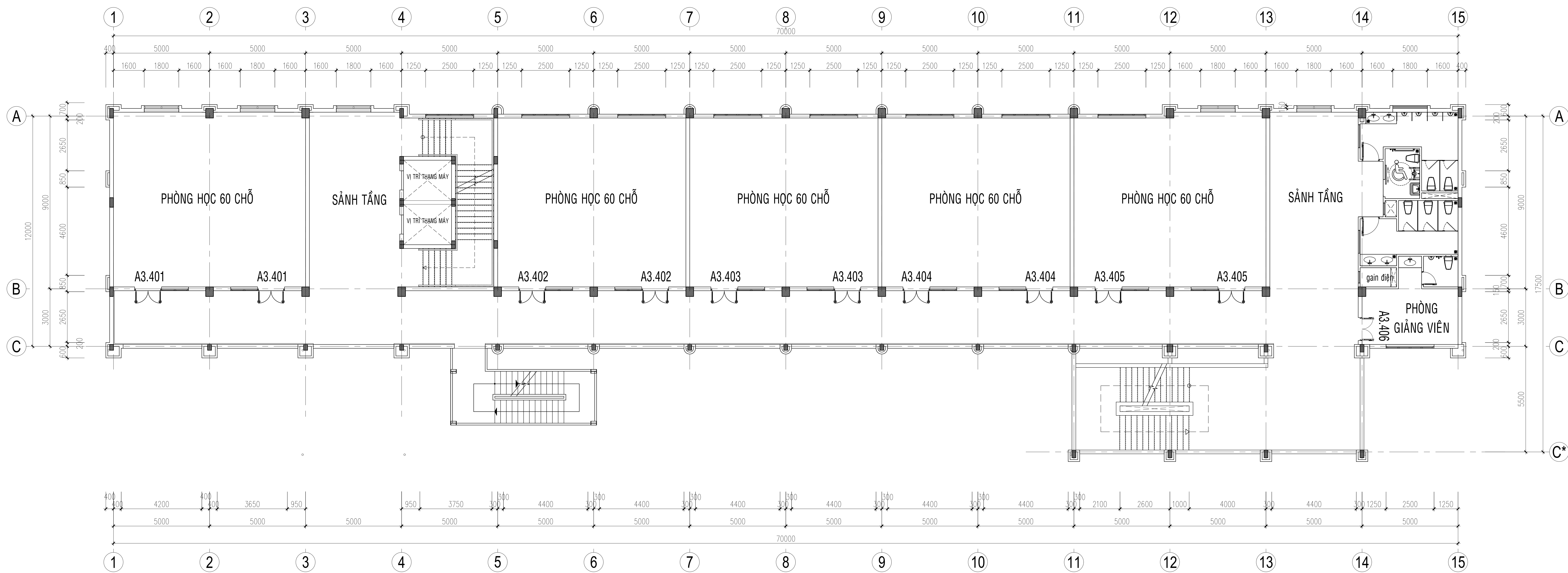
MẶT BẰNG BỐ TRÍ PHÒNG TẦNG 4
