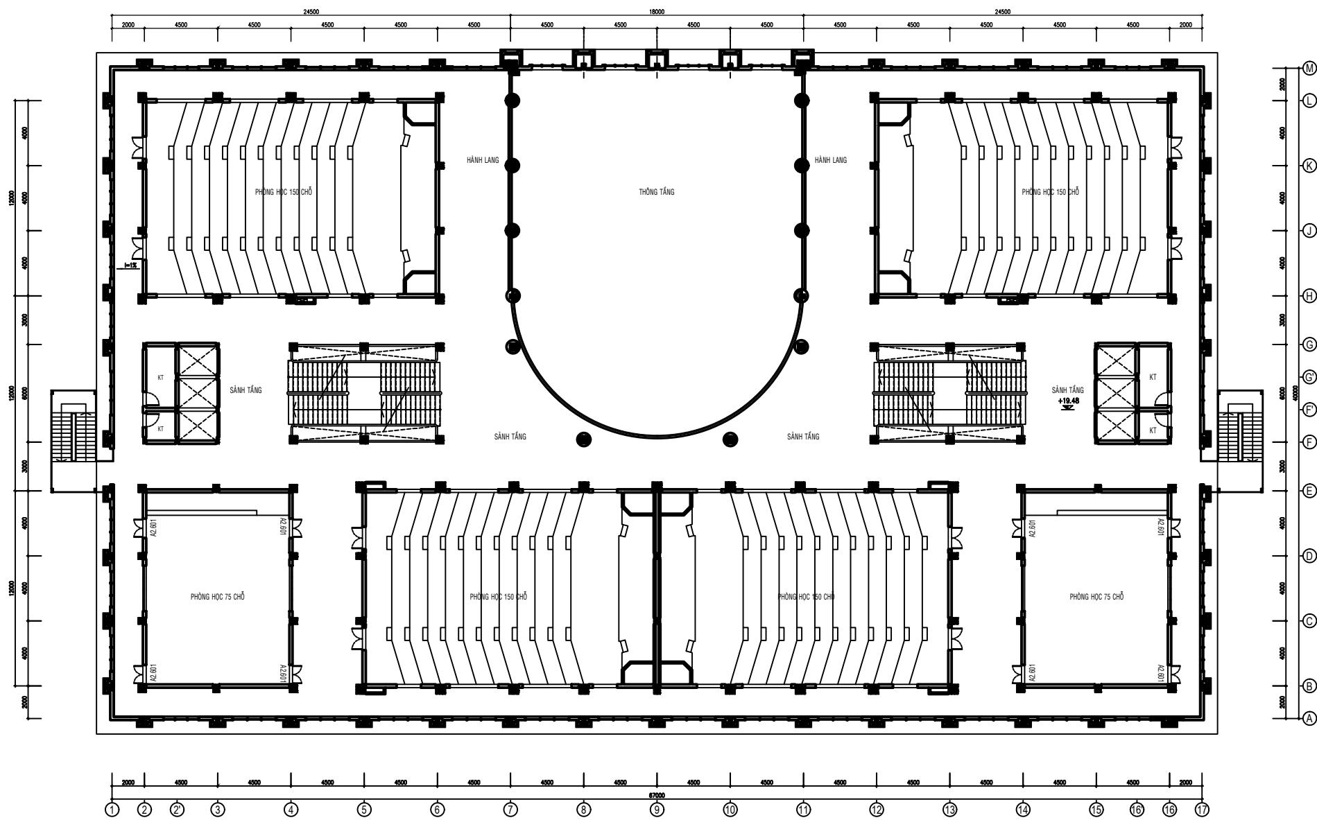
MẶT BẰNG BỐ TRÍ PHÒNG TẦNG 6 (TỶ LỆ : 1/100)
